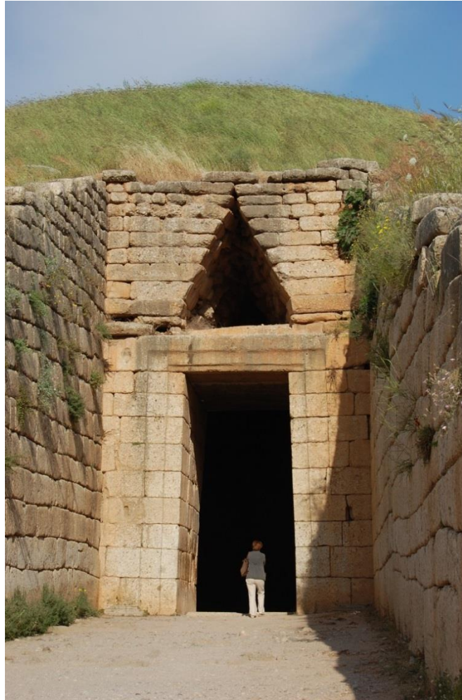
I Mykene leder en dromos (en muromgärdad lång gång) fram till Atreus kupolgrav. Kupolen bildas genom överkragning av överliggande stenskikt.
